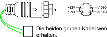
Kamerabuchse: Anschlußbelegung
